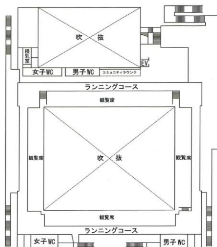
◆2階平面図
